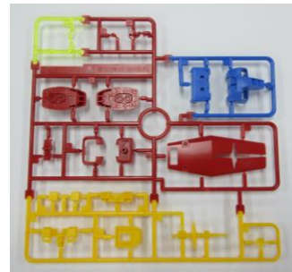
多色成形機で4色成形したランナー
